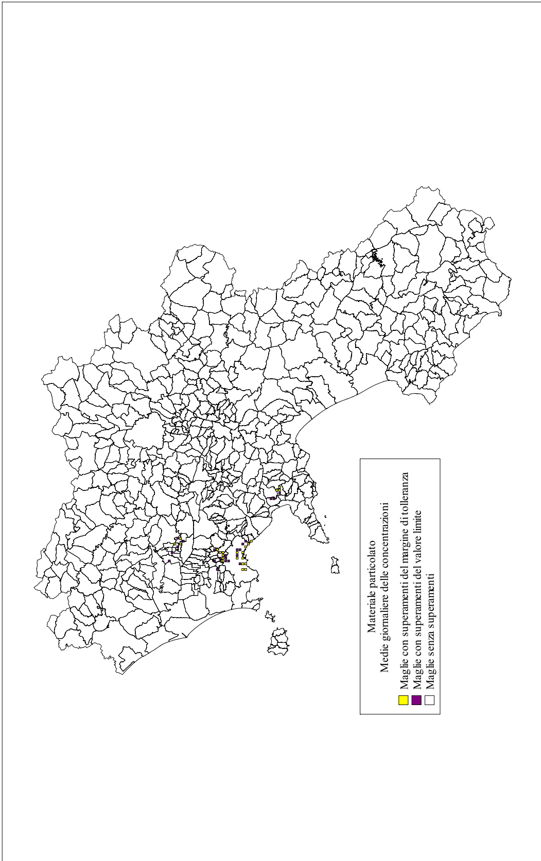
Figura 4 - Maglie critiche con riferimento al limite giornaliero per le PM_{10}
