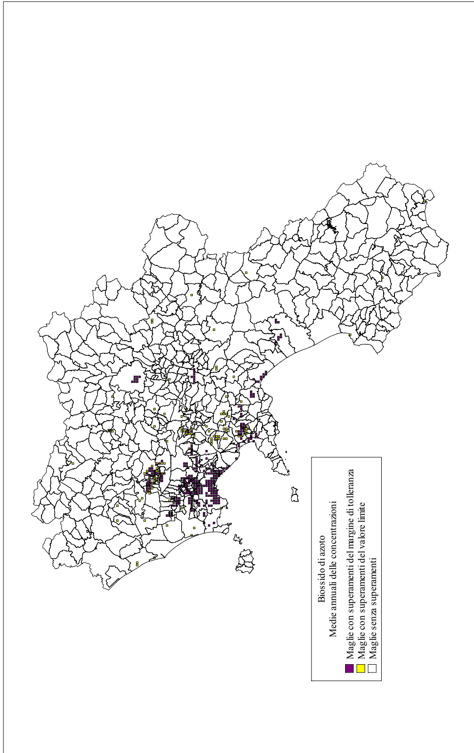
Figura 3 – Media annuale delle concentrazioni di biossido di azoto stimate per maglia
